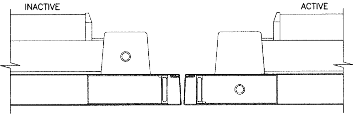
MTG. STILES DOUBLE DOOR
