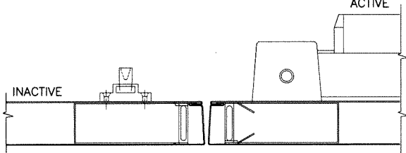
MTG. STILES DOUBLE DOOR
